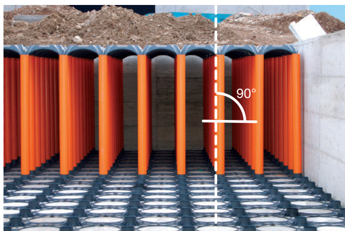
Sistema Nuovo Elevator Tank con griglia Quatro
