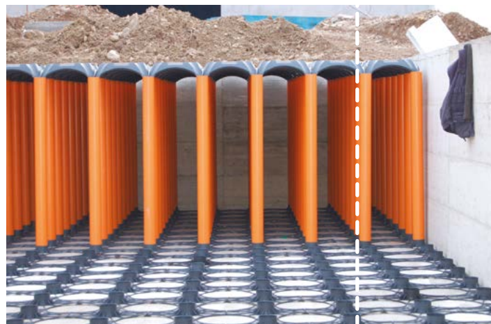
Système Nouveau Elevetor Tank avec grille
