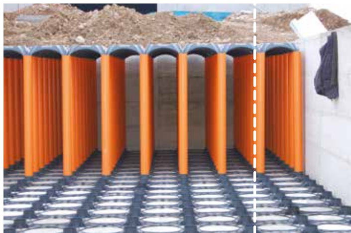
Sistema Nuevo Elevetor Tank con grilla
