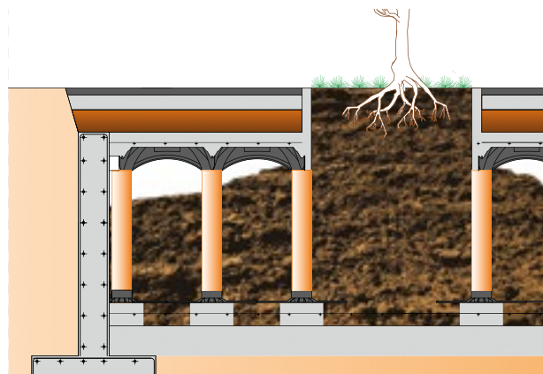
Sección sistema Nuevo Elevetor
