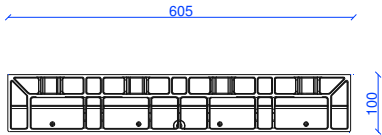
VISTA ESTERNA
