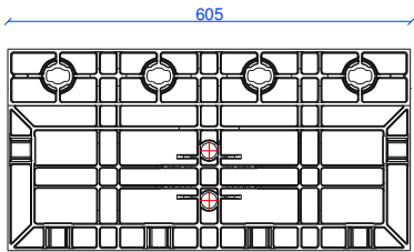
VUE EXTÉRIEURE
