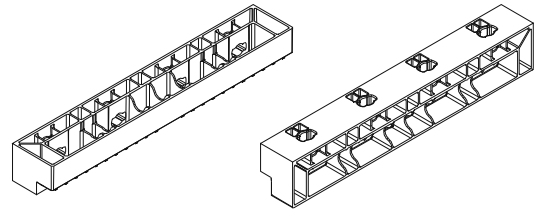
VUE AXONOMÉTRIQUE EXTERNE
