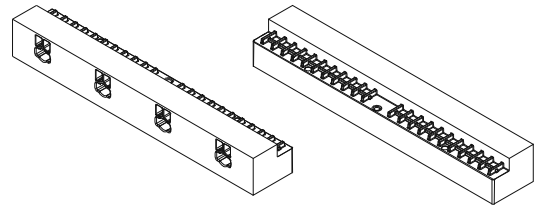
VUE AXONOMÉTRIQUE INTERNE
