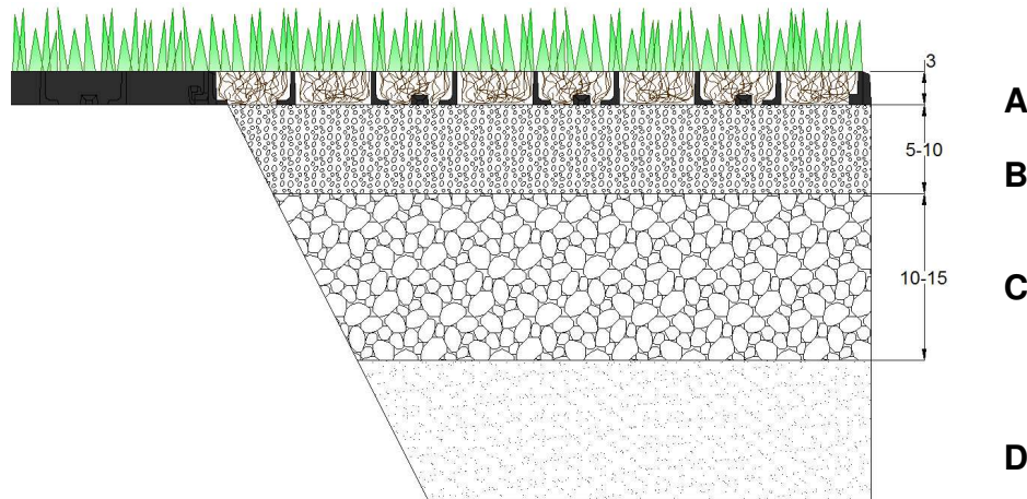
A- Runfloor F03; B- Strato di allettamento; C- Strato portante; D- Terreno naturale
