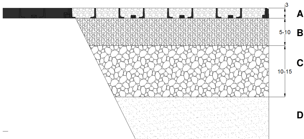
A- Runfloor F04; B- Strato di allettamento; C- Strato portante; D- Terreno naturale
