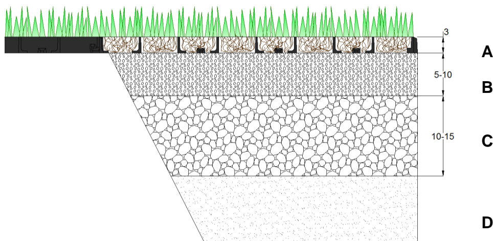
A - Runfloor 40 - H05; B - Strato di allettamento; C - Strato portante; D - Terreno naturale
