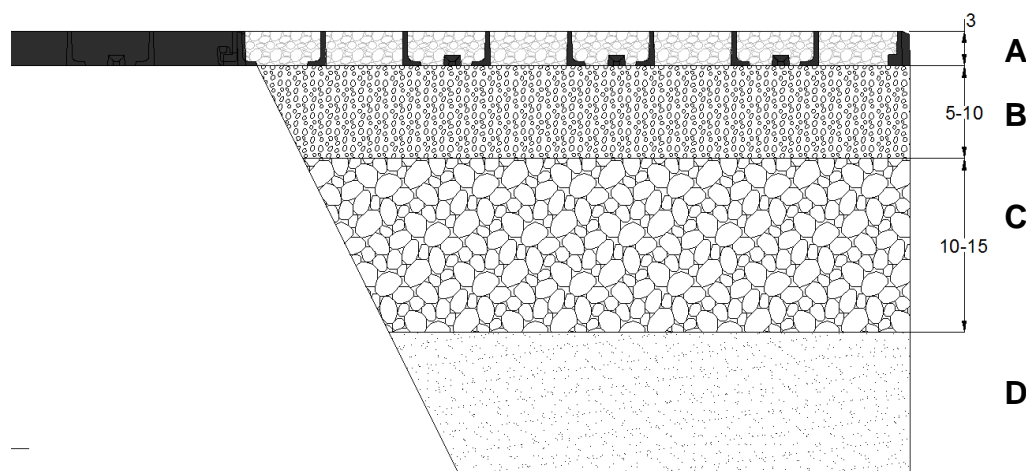
A - Runfloor 40 - H05; B - Strato di allettamento; C - Strato portante; D - Terreno naturale
