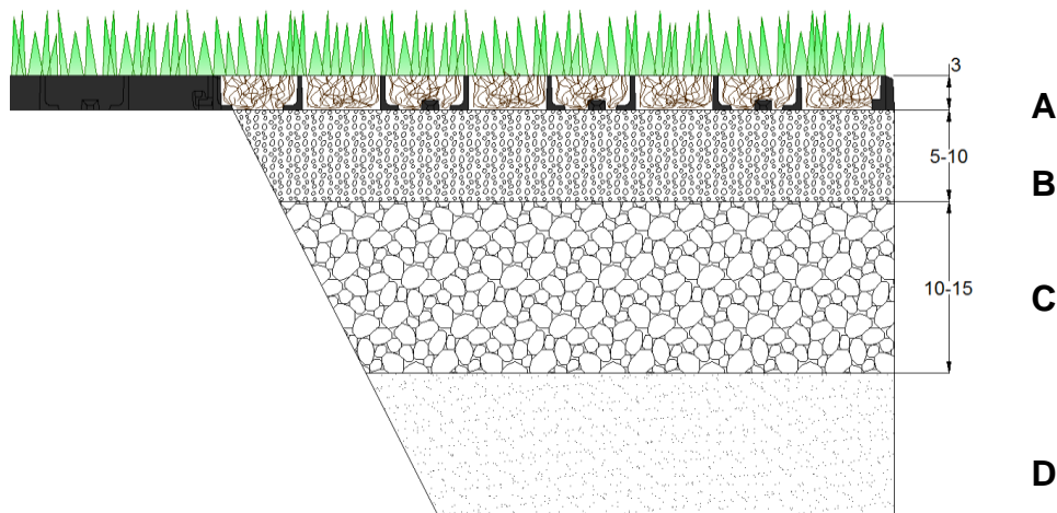
A - Runfloor 40-S05; B - Strato di allettamento; C - Strato portante; D - Terreno naturale
