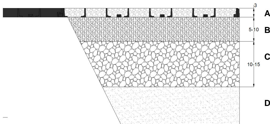
A - Runfloor 40 - S05; B - Strato di allettamento; C - Strato portante; D - Terreno naturale
