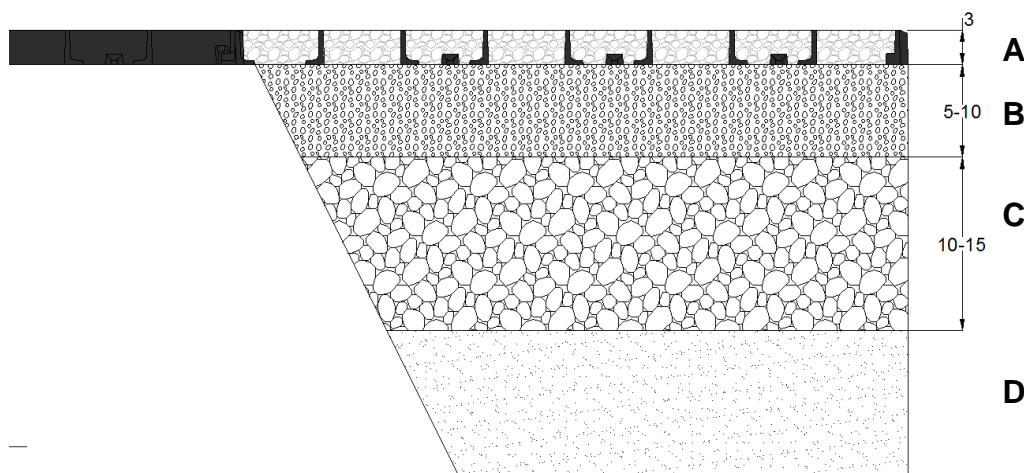
A- Runfloor F03; B- Strato di allettamento; C- Strato portante; D- Terreno naturale
